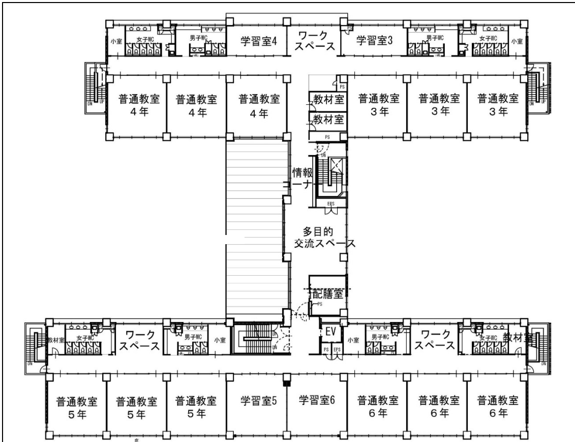
3階平面図
