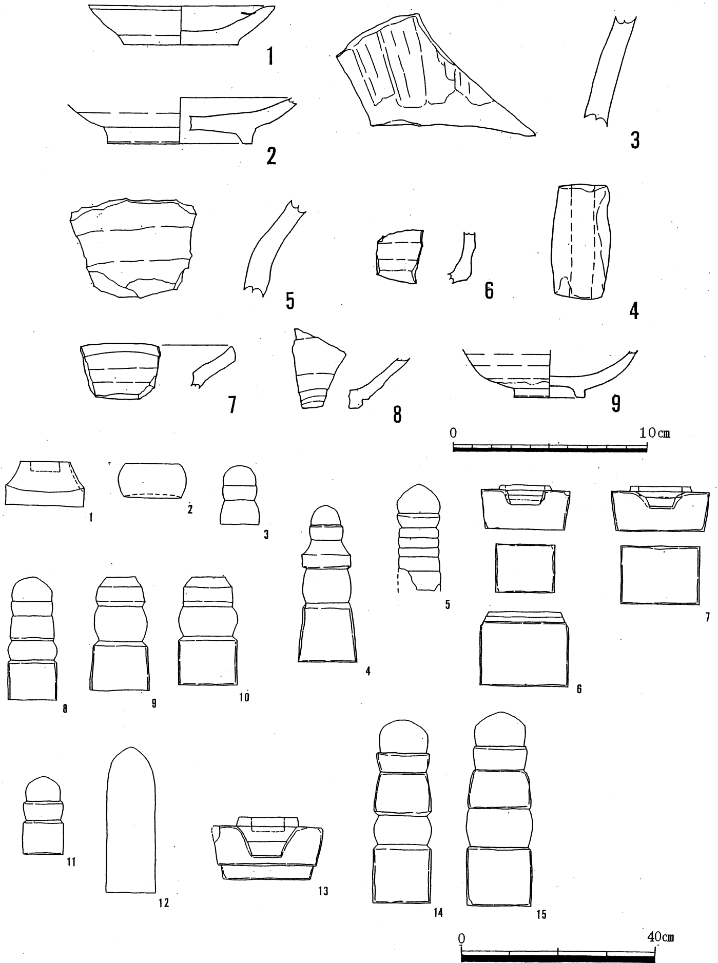
第4図 遺物・石塔実測図
